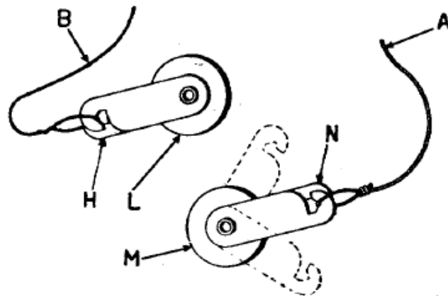
PHONOLA RADIO - Modelli 417-575-579-579 A-580 - Montaggio funicella della scala parlante.
